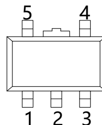
SOT-89-5L
